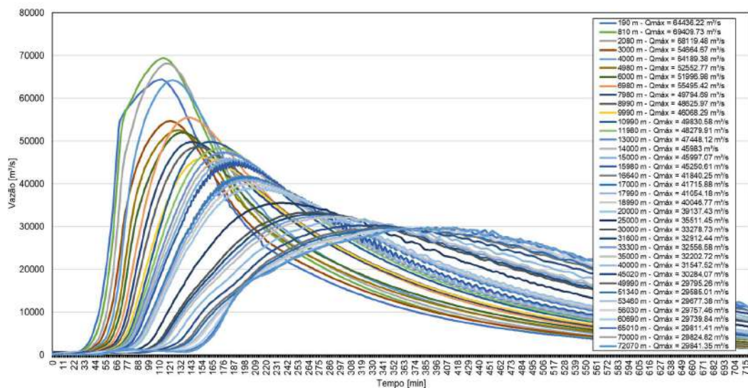
Figura 15- Propagação de hidrogramas nas seções de controle. RDC 1.
