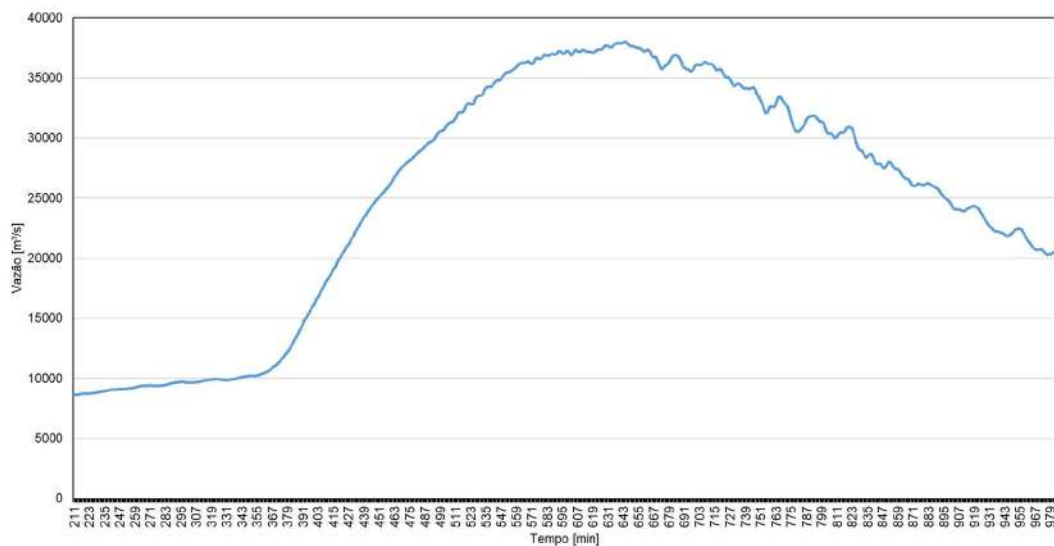
Figura 23. Hidrograma de ruptura na entrada do reservatório da UHE Itumbiara - RSC 1.
