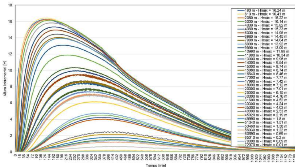
Figura 17. Altura incremental da onda propagada nas seções de controle. RDC 3.
