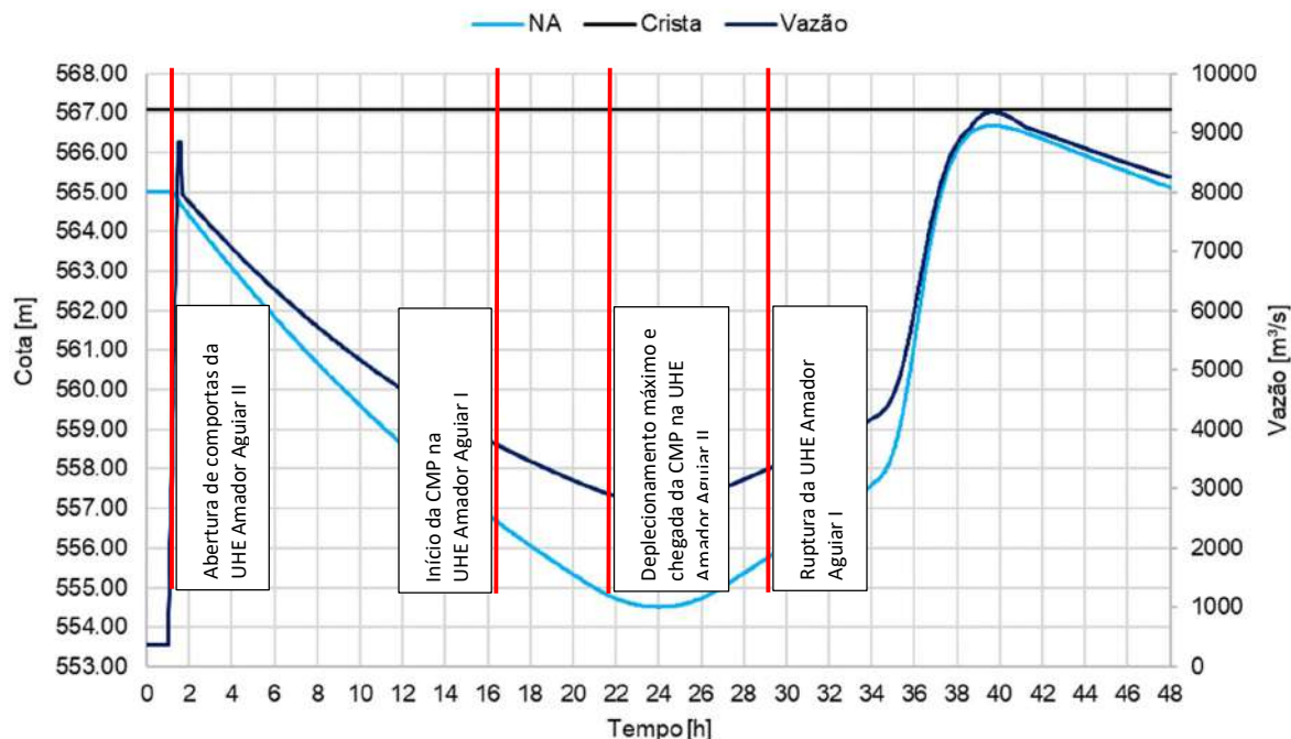
Figura 14. Operação para amortecimento na UHE Amador Aguiar II da onda de ruptura do cenário RDC 4 da UHE amador Aguiar I.
