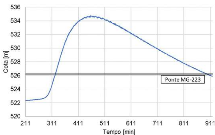
Figura 28. Cotagrama da ponte rodovia MG-223 - RSC 1.
