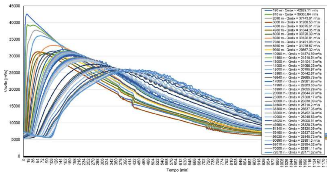
Figura 4. Propagação de hidrogramas nas seções de controle. RDC 3.
