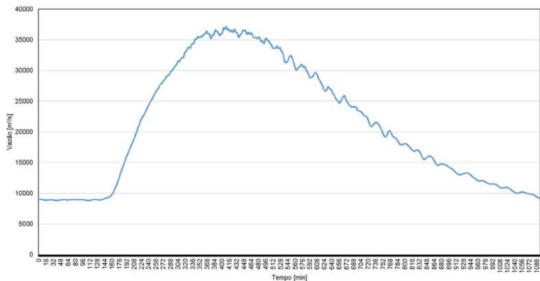
Figura 5. Hidrograma de ruptura na entrada do reservatório da UHE Itumbiara - RDC 2.
