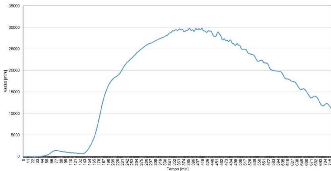
Figura 20. Hidrograma de ruptura na entrada do reservatório da UHE Itumbiara - RDC 1.
