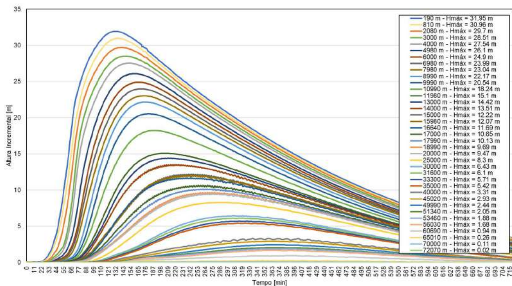
Figura 16. Altura incremental da onda propagada nas seções de controle. RDC 1.
