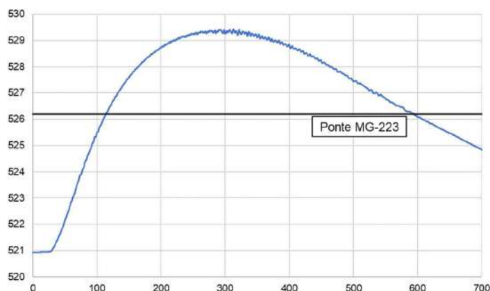
Figura 27. Cotagrama da ponte rodovia MG-223 - RDC 3.
