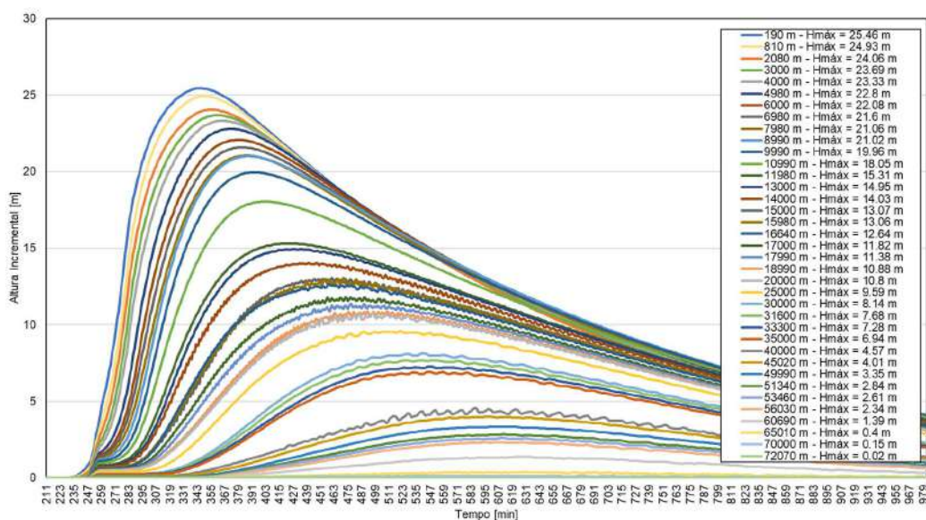
Figura 19. Altura da onda propagada nas seções de controle. RSC 1.
