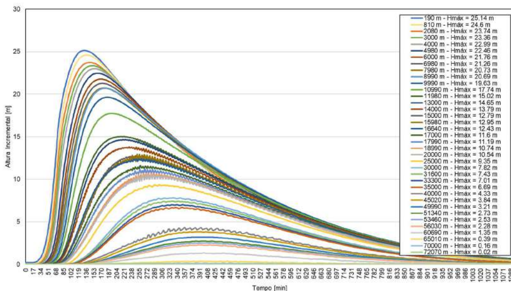
Figura 18. Altura da onda propagada nas seções de controle. RDC 2.
