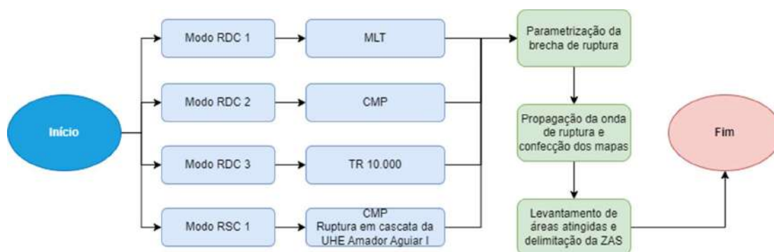
Figura 122. Cenários de ruptura da UHE Amador Aguiar II.
