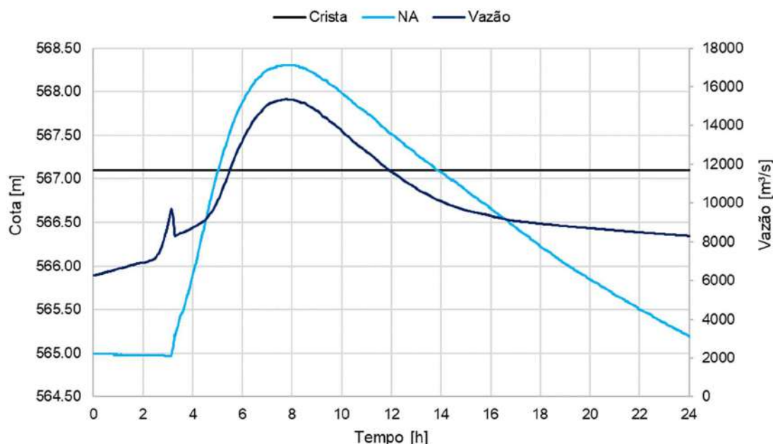
Figura 3. Hidrograma e cotagrama de ruptura da UHE Amador Aguiar I na seção da UHE Amador Aguiar II – RDC 4.
