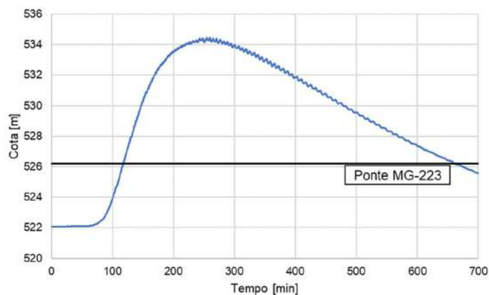
Figura 26. Cotagrama da ponte rodovia MG-223 - RDC 2.
