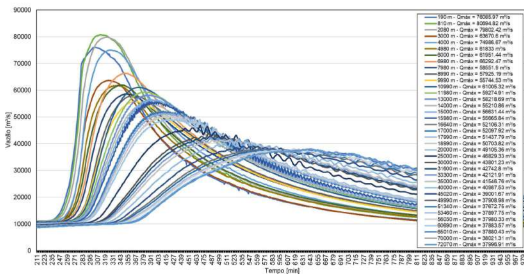
Figura 18. Propagação de hidrogramas nas seções de controle. RSC 1.
