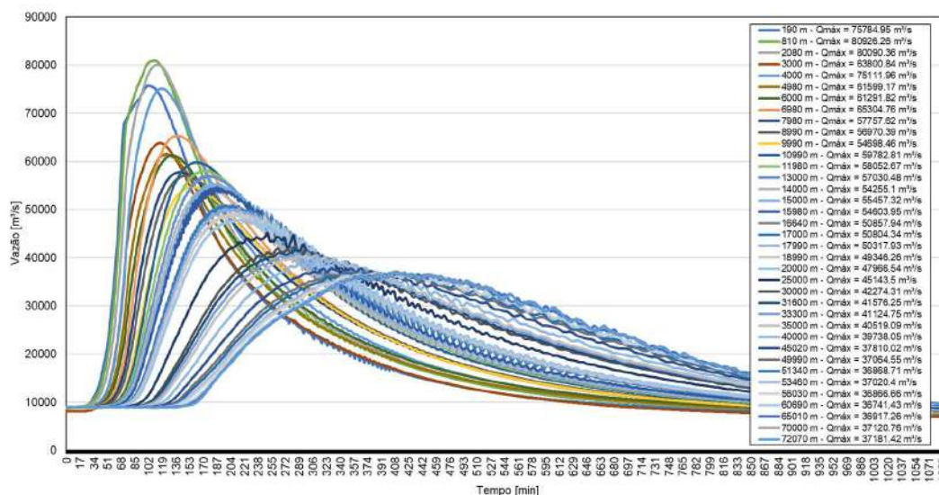
Figura 17. Propagação de hidrogramas nas seções de controle. RDC 2.
