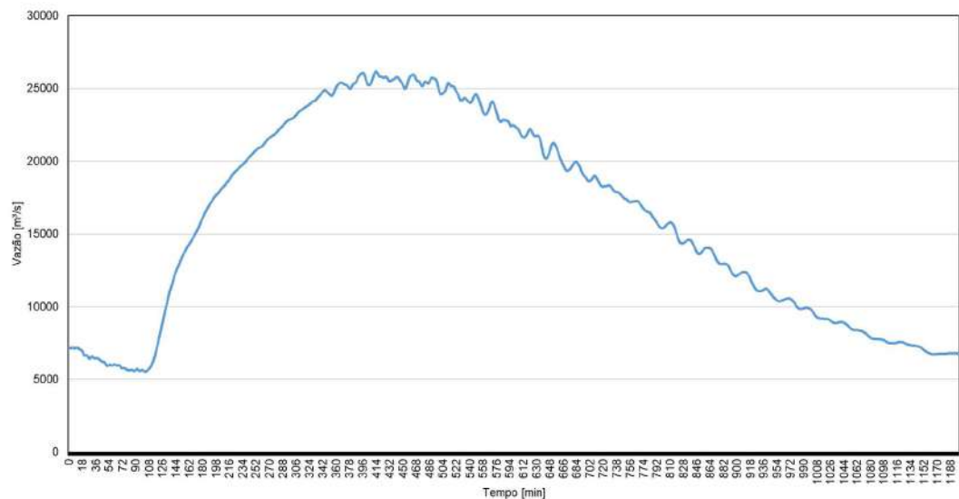
Figura 22. Hidrograma de ruptura na entrada do reservatório da UHE Itumbiara - RDC 3.
