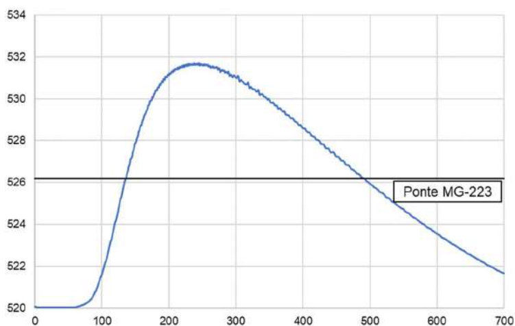
Figura 25. Cotagrama da ponte rodovia MG-223 - RDC 1.
