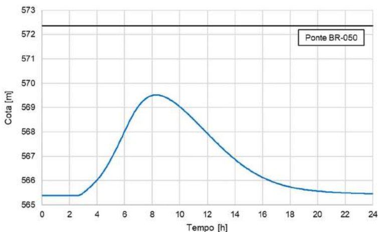
Figura 29. Cotagrama da ponte rodovia BR-050 - RDC 3.
