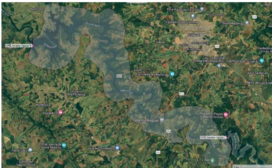
Figura 11- Modelo HEC-RAS.
