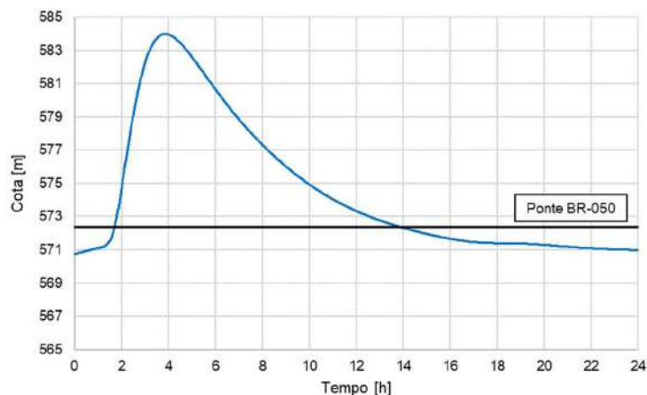
Figura 30 . Cotagrama da ponte rodovia BR-050 - RDC 4.
