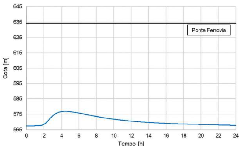
Figura 34. Cotagrama da ponte ferrovia Pontilhão do A - RDC 4.
