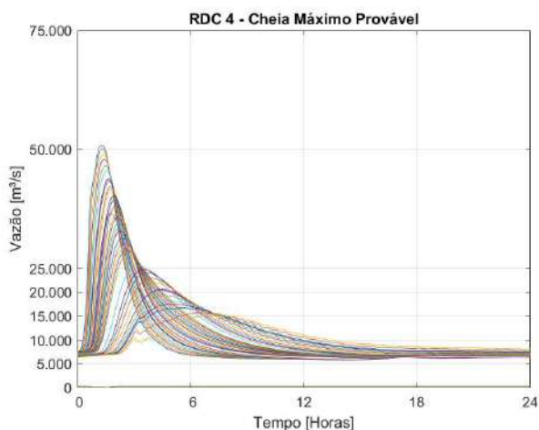
Figura 22 Propagação de hidrogramas nas seções de controle. RDC 4.
