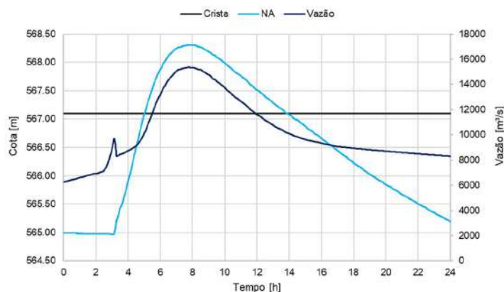
Figura 24. Hidrograma e cotagrama da onda de ruptura na UHE Amador Aguiar II (RDC 4).
